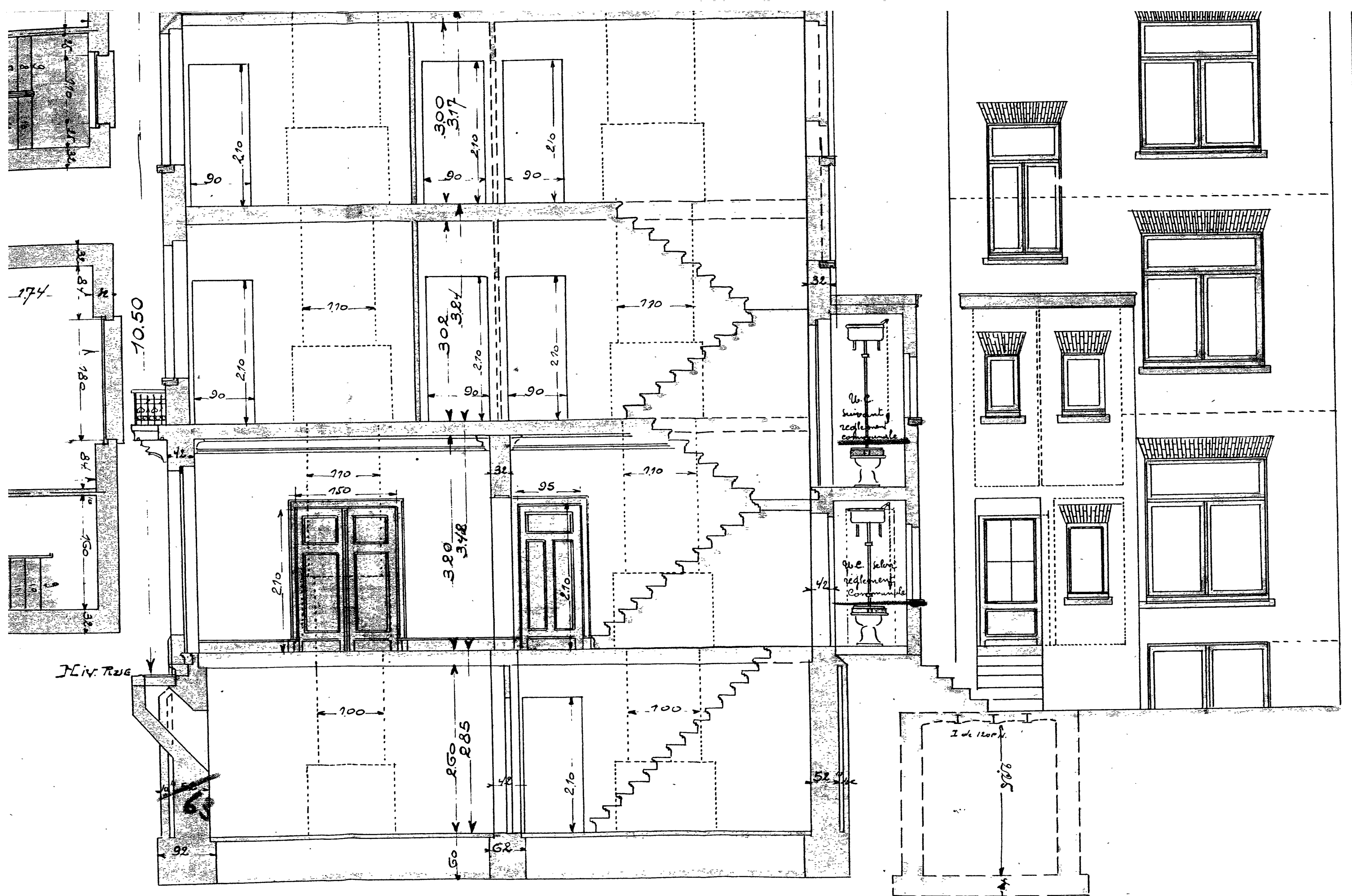
COUPE LONGITUDINALE
